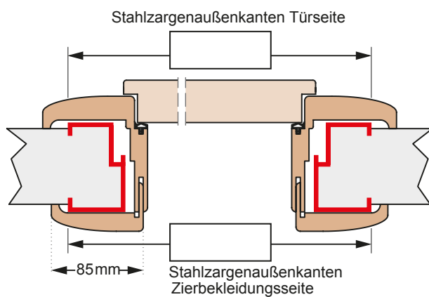
Renovierzarge 04 bombiert
