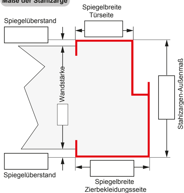
Maße der Stahlzarge
