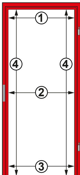
Lichte Durchgangsmaße der Stahlzarge
